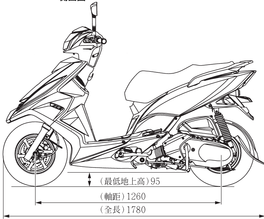
側面圖
