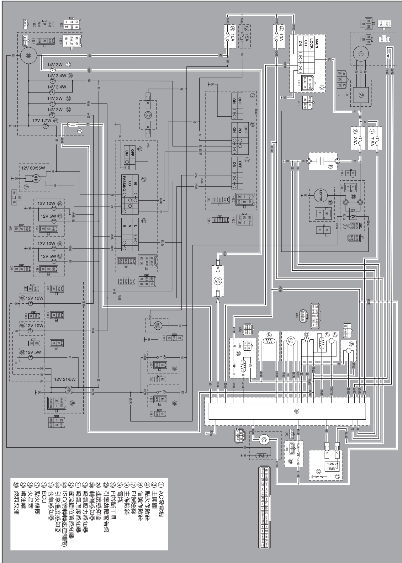
線路圖(17C1)
